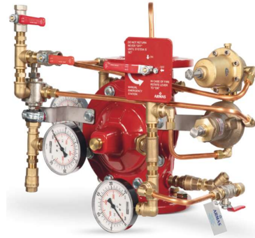
77DE-PORV-PR-MR Manuel Reset
